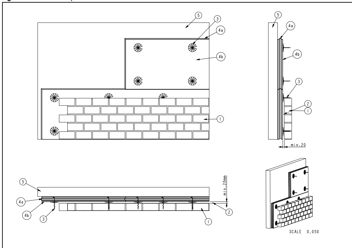
Figuur 2 – Constructieopbouw 2.
