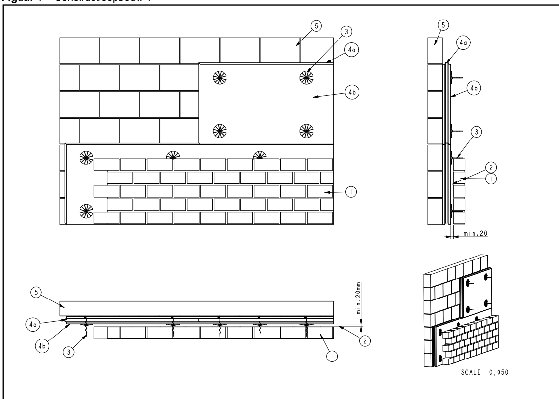
Figuur 1 – Constructieopbouw 1
