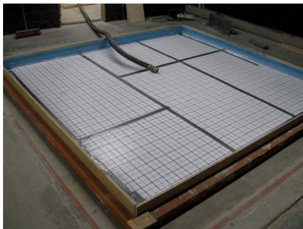
Isomo isolatieplaten, naden afgetaped
